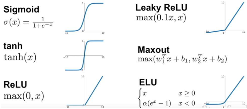
Şekil 5.5. Yapay sinir ağlarında sıklıkla kullanılan aktivasyon fonksiyonları
