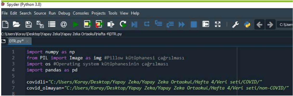
Şekil 4.4. Gerekli kütüphaneleri ve komutların kod gösterimi
