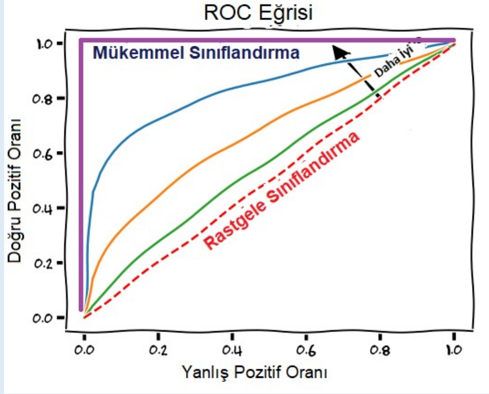
Şekil 4.12. ROC Eğrisi gösterimi
