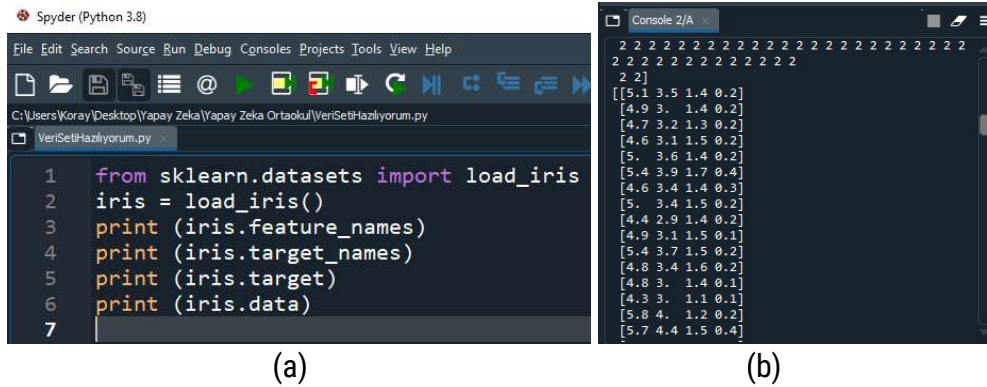
Şekil 1.19. Veri analizi a) bağımsız değişkenleri sayısallaştırma kodu b) görüntüsü
