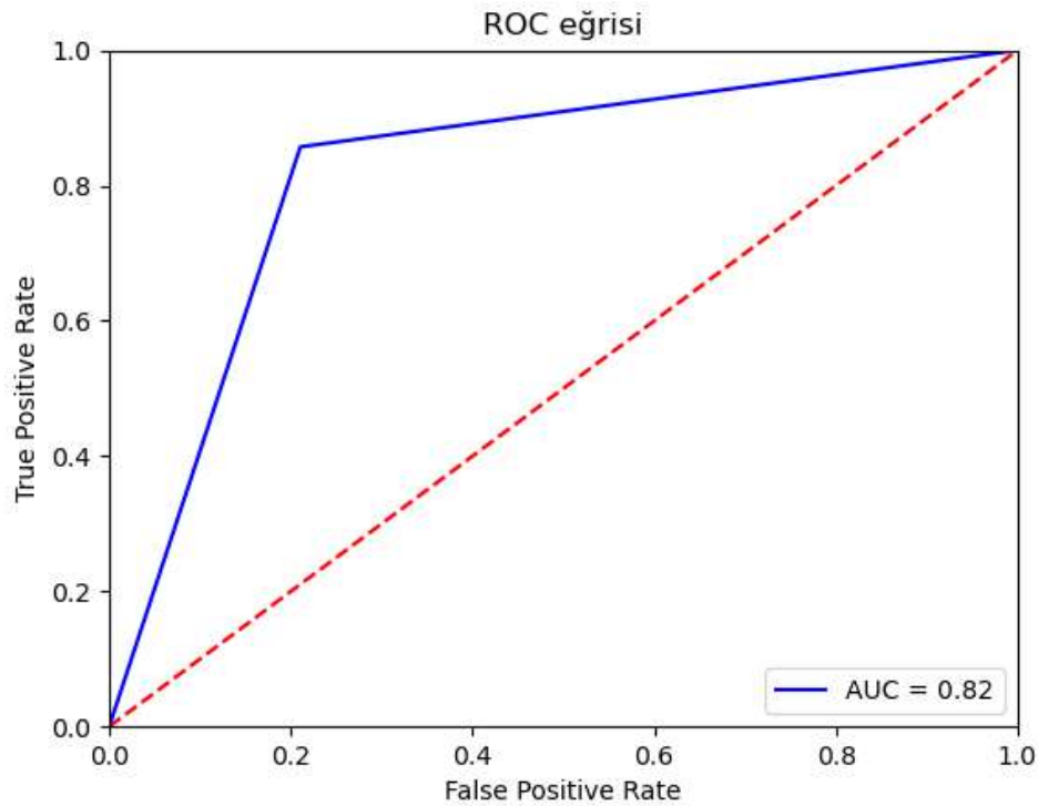
Şekil 4.21. Elde edilen ROC eğrisi
