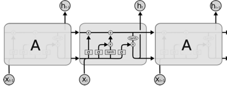
Şekil 8.5. LSTM Network Yapısı (Web Kaynağı 8.4)
