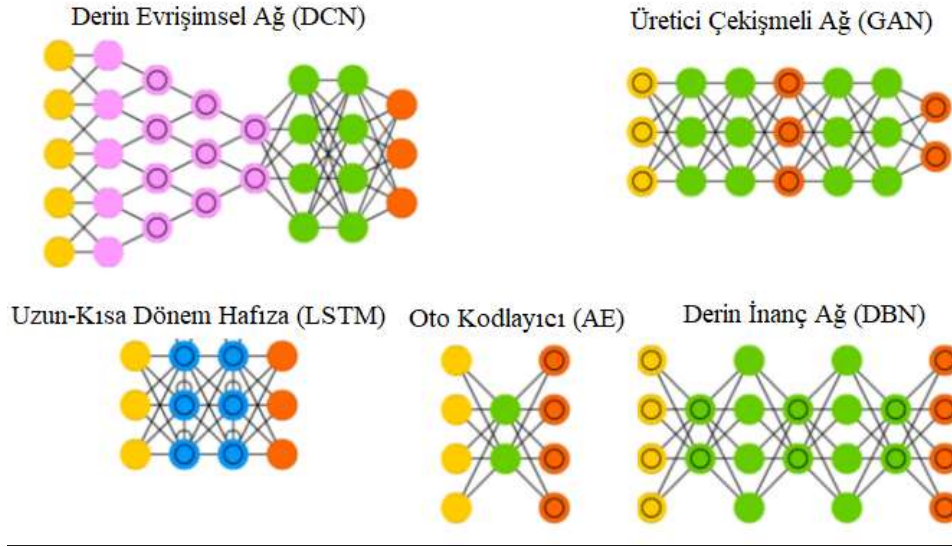
Şekil 8.2. Derin öğrenme mimarileri (Web Kaynağı 8.1)
