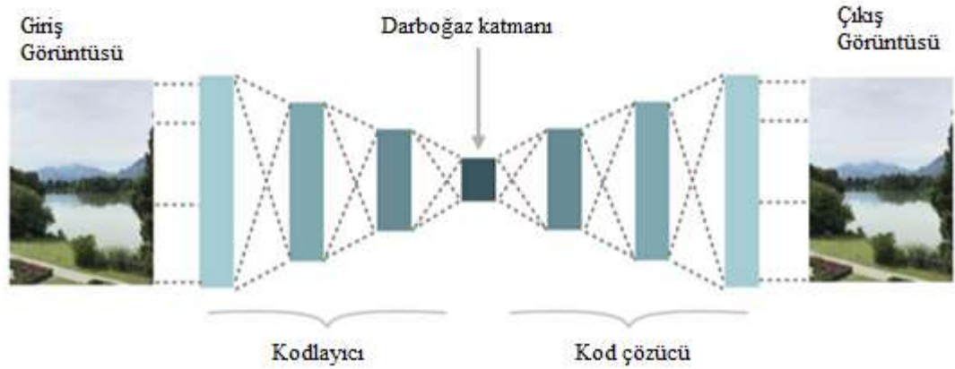
Şekil 8.6. Oto kodlayıcı tekniği şematiği (Web Kaynağı 8.5)
