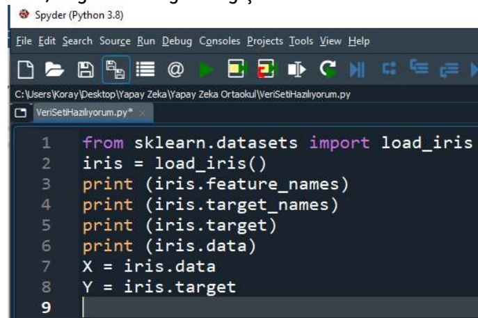
Şekil 1.20. Bağımlı ve bağımsız değişkenleri X ve Y değişkenine atama kod satırı
