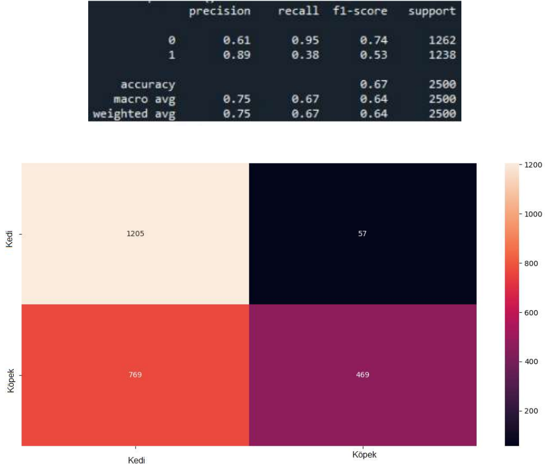
Şekil 8.15. Karmaşıklık matrisi görüntülemeleri
