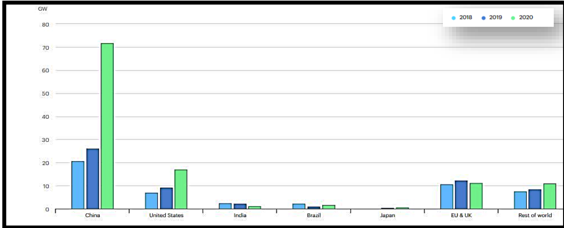
Şekil 8-4 Dnya yıllık rzgr kapasitesi ilaveleri¹⁸
