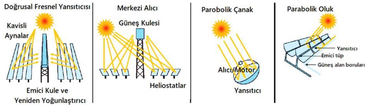
Şekil 6-2 CSP teknolojileri 14
