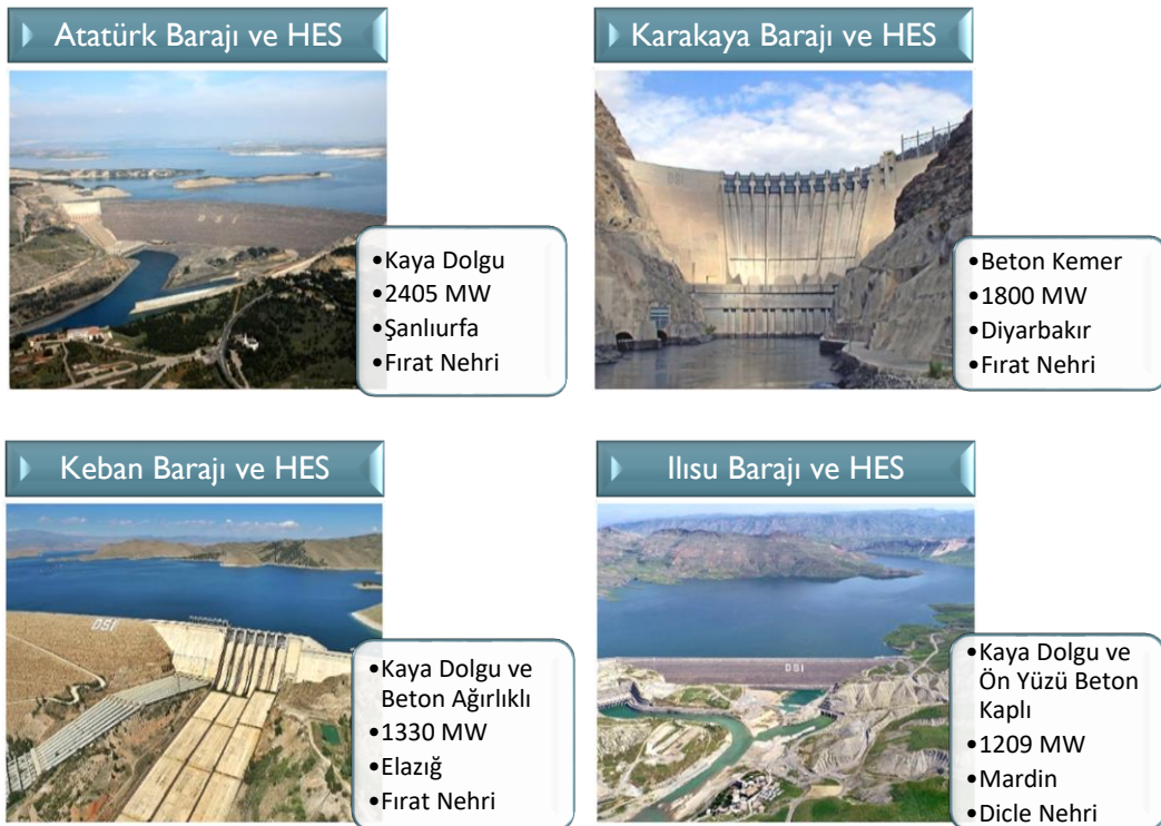
Şekil 5-2 Türkiye’nin en büyük dört hidroelektrik santralleri 13
