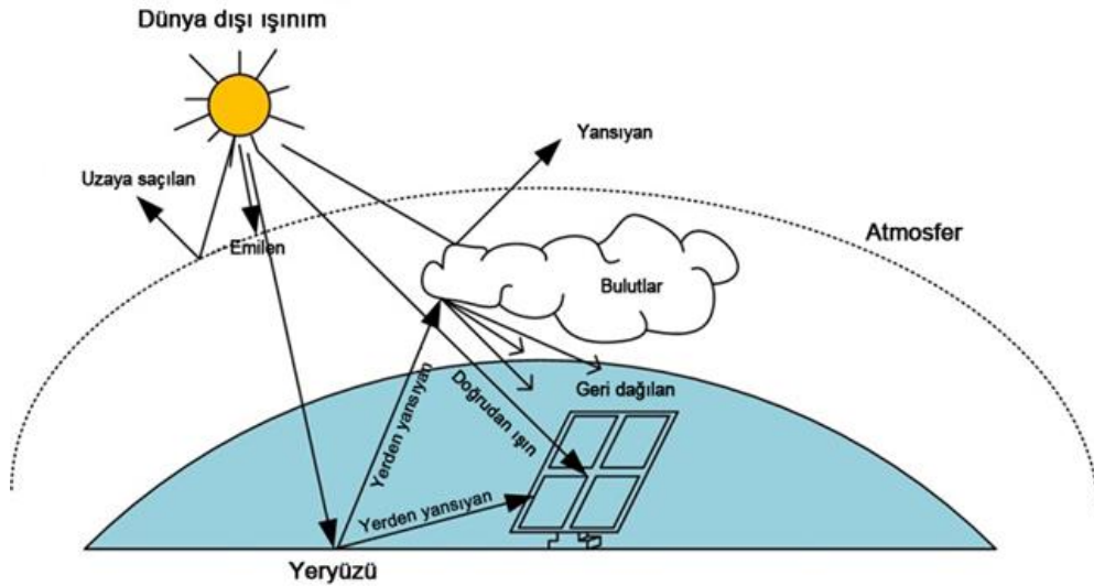
Şekil 6-1 Atmosfer ve yüzey tarafından ayrılmış Güneş ışıınını bileşenleri
